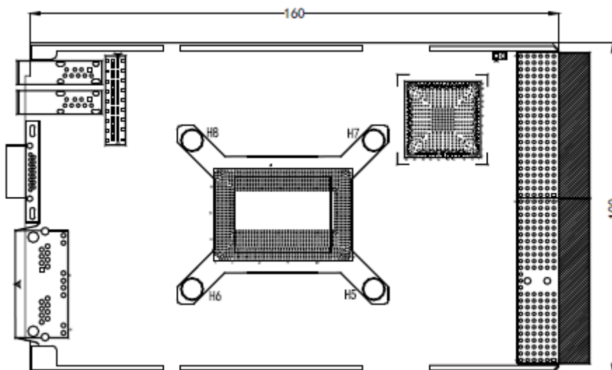
CPC-3816B-MB
